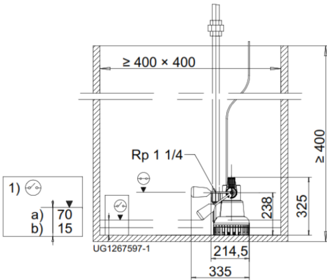
Abb. 3: Abmessungen AmaDrainer 301
