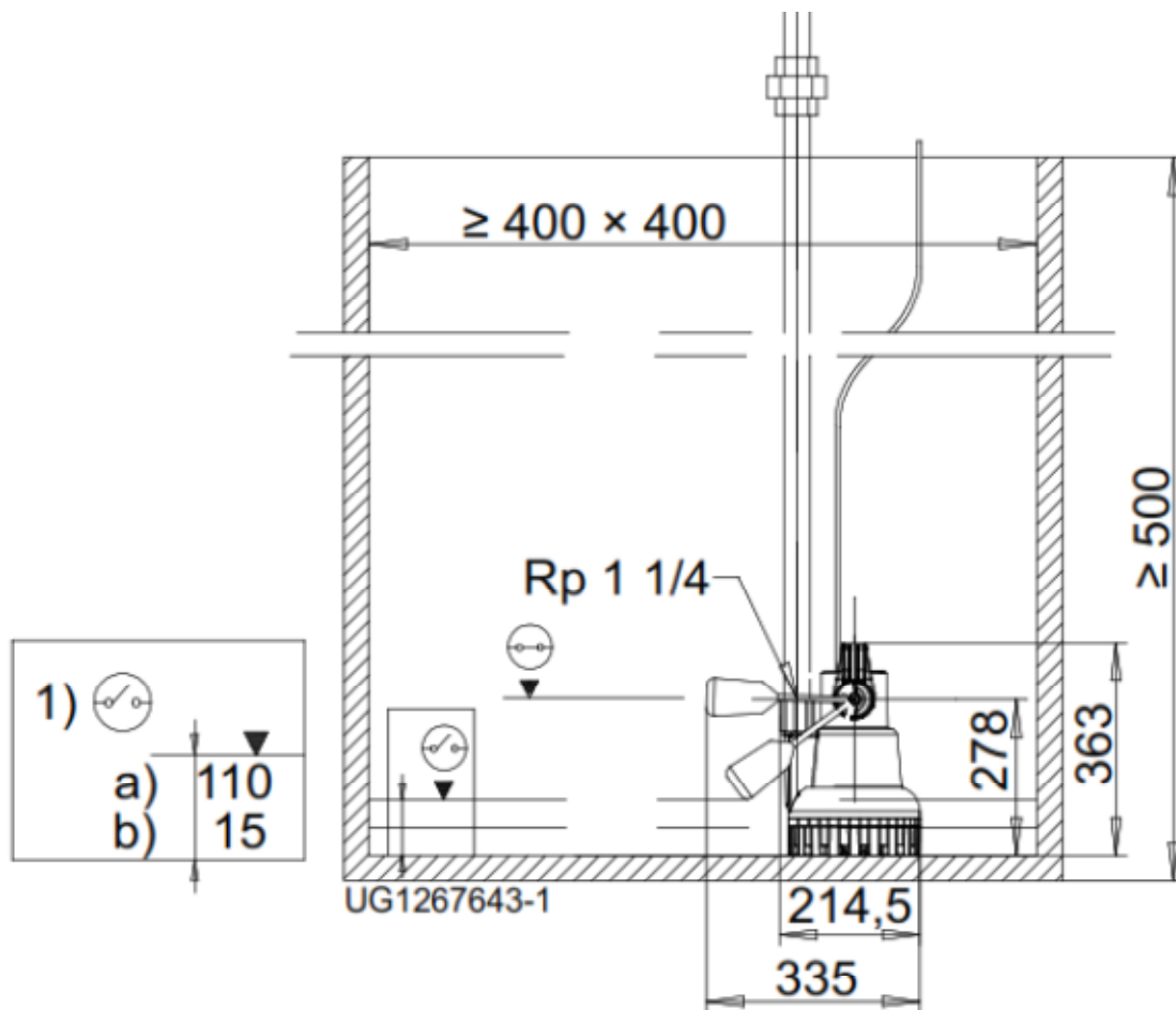
Abb. 4: Abmessungen AmaDrainer 302/303
