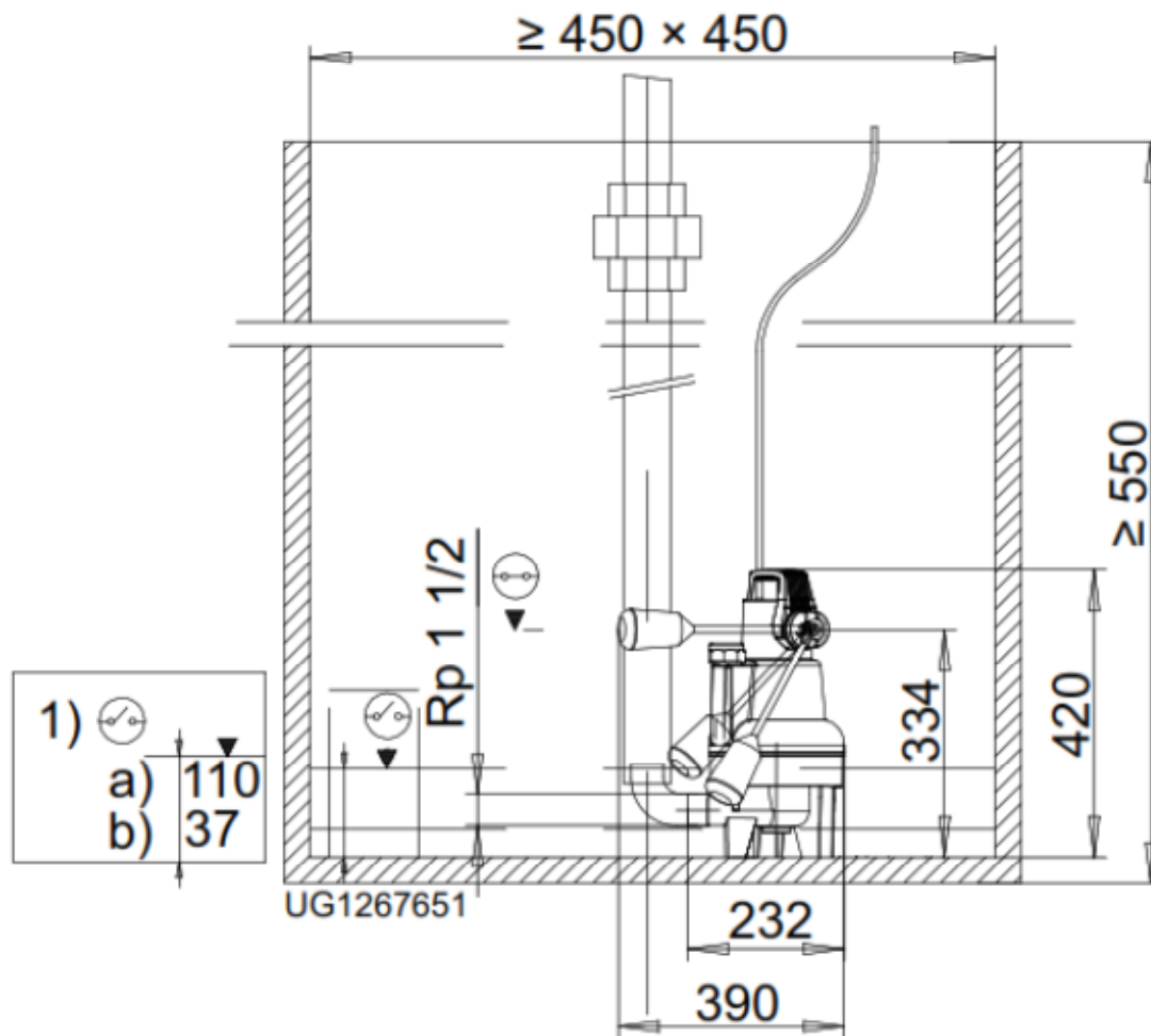
Abb. 5: Abmessungen AmaDrainer 358
