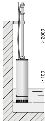
Abb. 3: Pumpenaggregat auf Boden stehend [mm]
