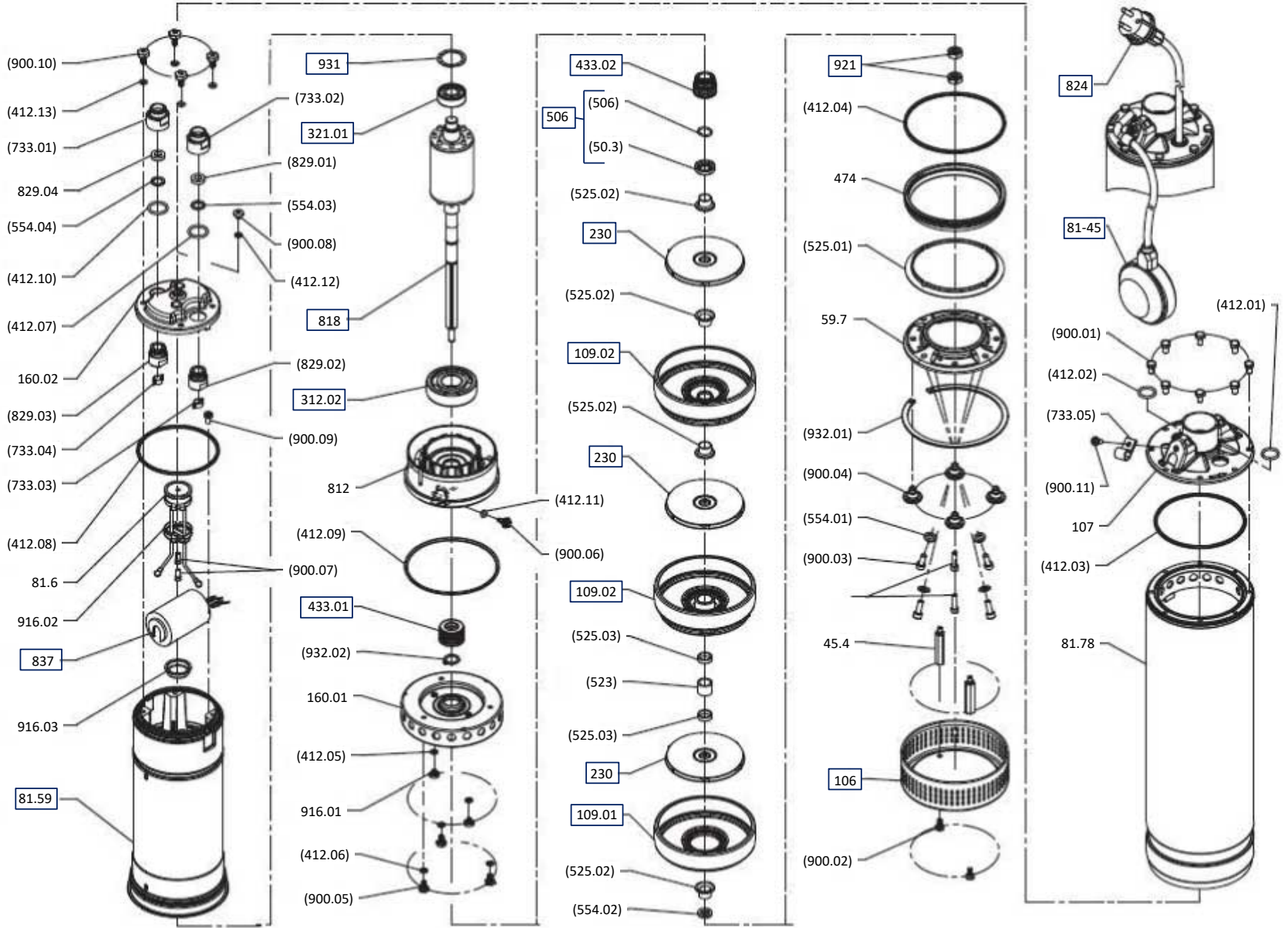
Abb. 7: Explosionszeichnung
